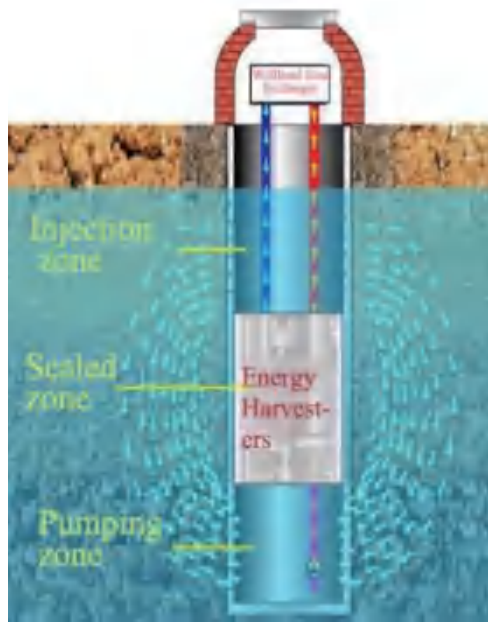
无传热回填型
