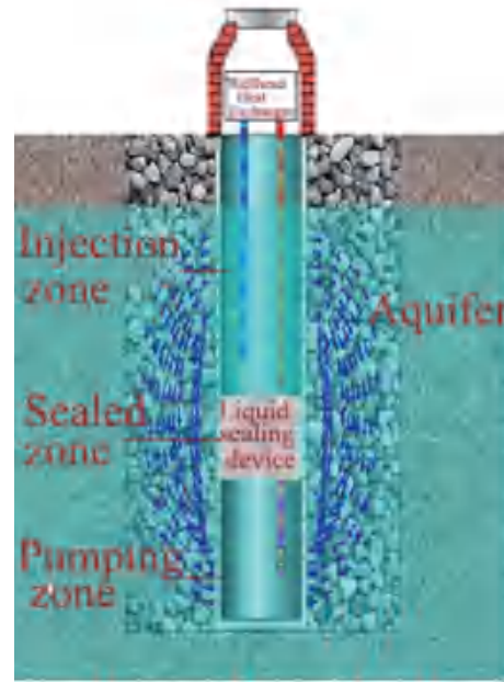
有传热回填型
